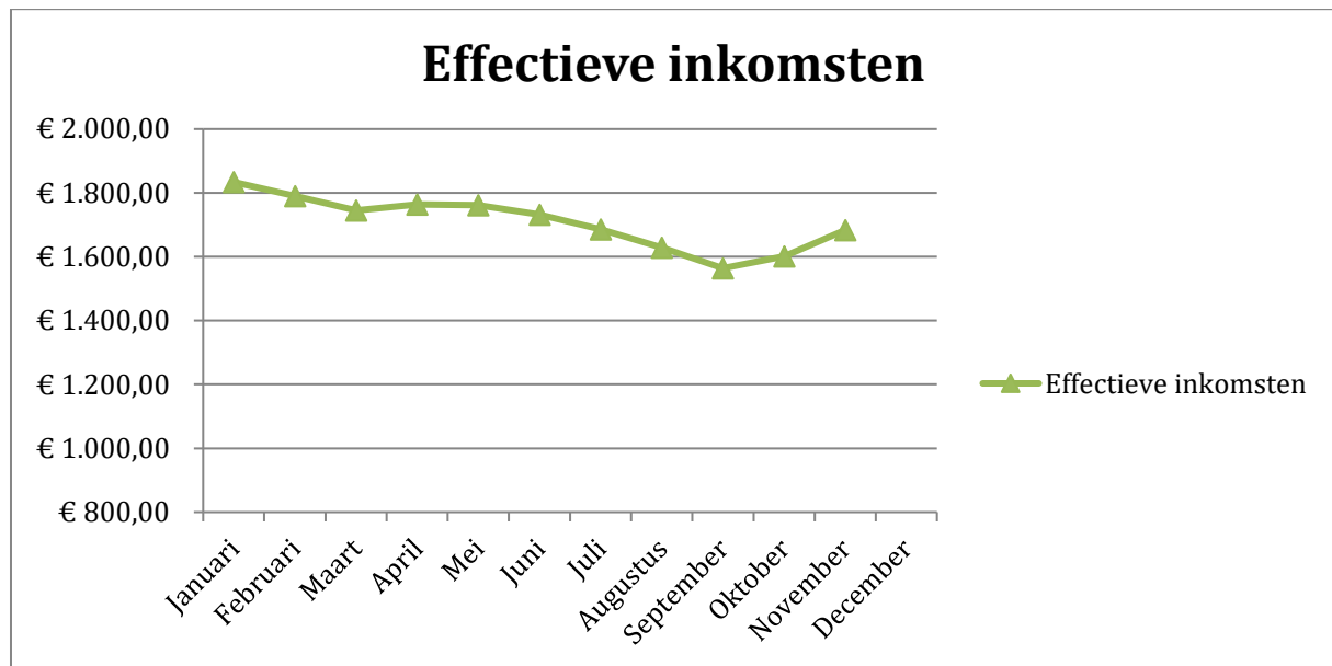
Grafiek 2. Maandelijke inkomsten van donateurs in het jaar 2018
