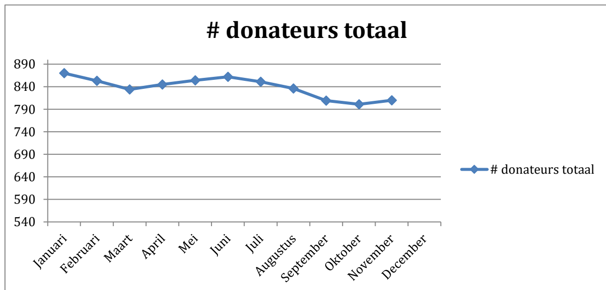
Grafiek 1. Aantal donateurs in 2019
